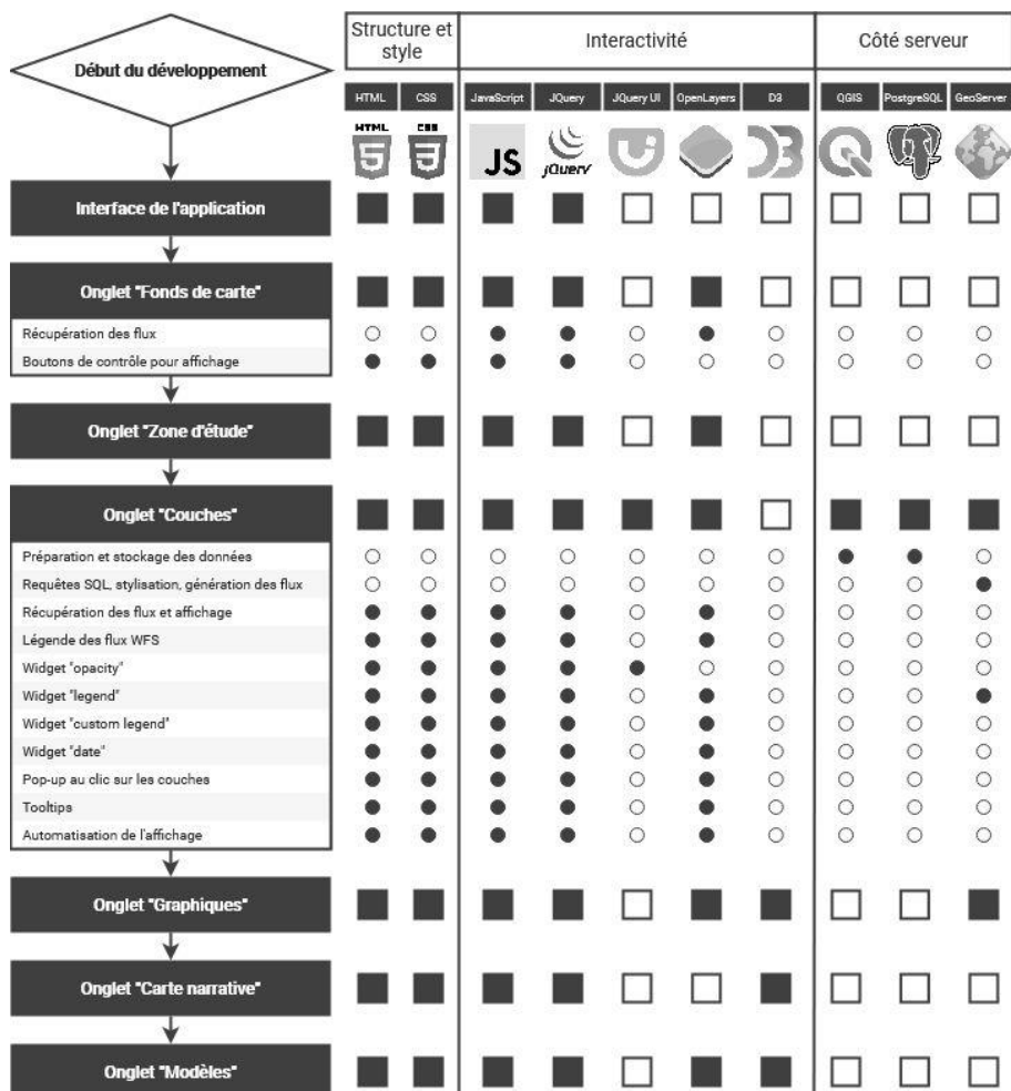
FIGURE 2. Principales étapes du développement de l'application et technologies mobilisées (source : auteurs)
