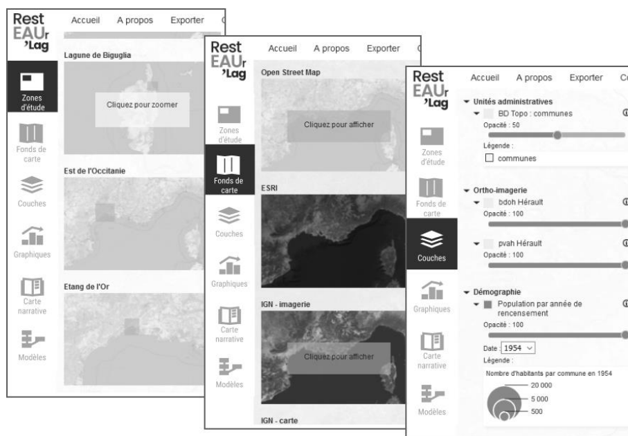
FIGURE 3. Principe multi-volets de l'interface géoweb du projet RestEAU'Ulag : les trois volets des zones d'études, des fonds de cartes et des couches géographiques (source : auteurs)
