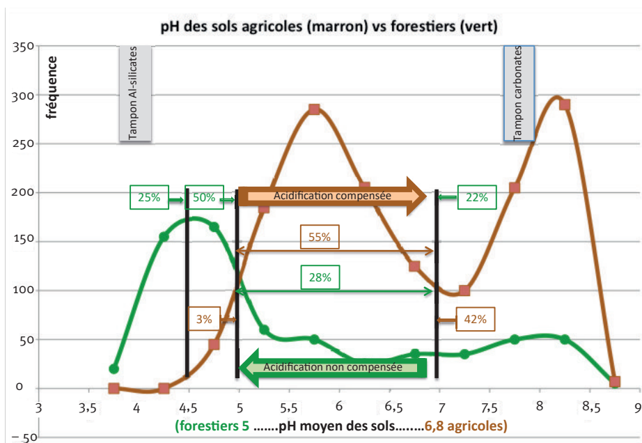
FIGURE 1 COMPARAISON DES SOLS AGRICOLES (courbe brune) ET FORESTIERS (courbe verte) POUR LEUR pH EAU Courbes établies à partir des données du RMQS (base de données GIS sols Inrae Infosol Orléans).
