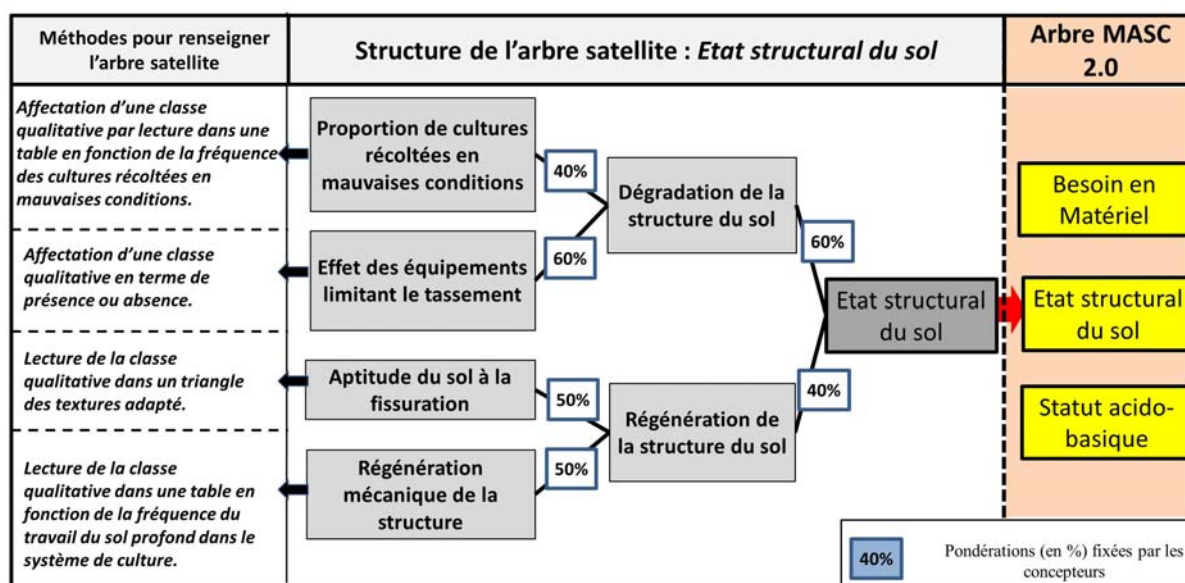
Figure 3 : Exemple d'un arbre satellite proposé dans MASC 2.0 pour renseigner le critère basique « Maîtrise de l'état structural du sol », appartenant à la dimension économique du développement durable).
