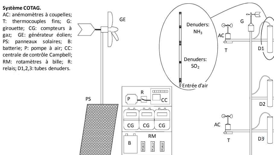
Figure M29.1. Système COTAG de (Famulari et al. , 2010)
