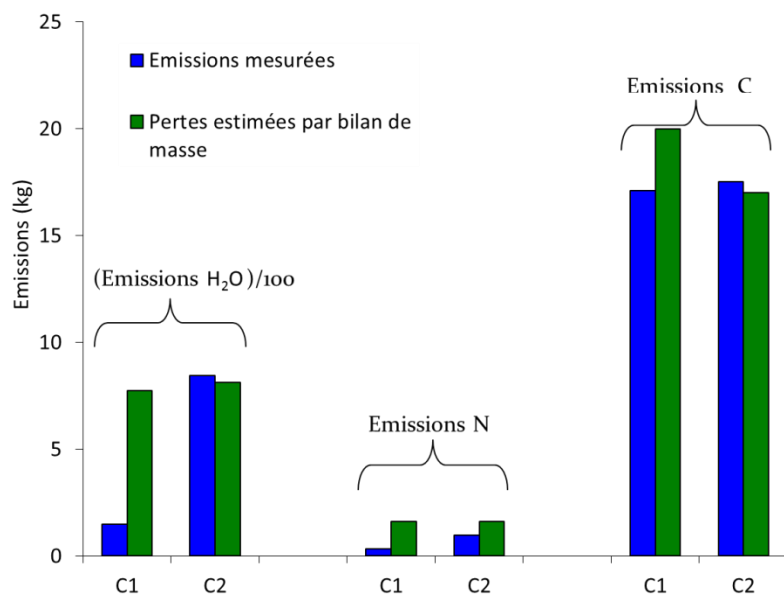
Figure C10.2. Emissions gazeuses (H 2 O, N, C) estimées à l'aide du bilan de masse et des systèmes de chambres dynamiques
