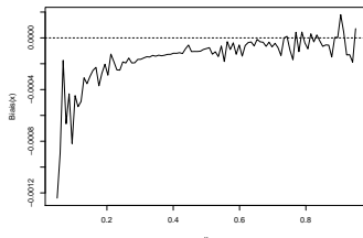
FIGURE 3.10 – Biais de -\hat{p}_s \ln \hat{p}_s entre 0 et 1.
