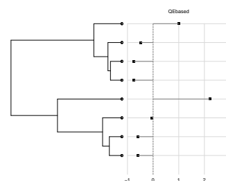
FIGURE 7.11 – Originalité des espèces.
