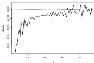
FIGURE 3.8 - Biais de -\hat{p}_s \ln \hat{p}_s entre 0 et 1.
