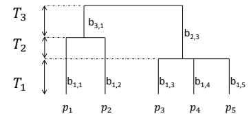
FIGURE 9.4 – Arbre phylogénétique ou fonctionnel hypothétique. Rappel de la figure 7.7(a). 5 espèces sont présentes ( S = 5 ), leurs probabilités notées p_1 à p_5 . Les noms des branches sont affichés.
