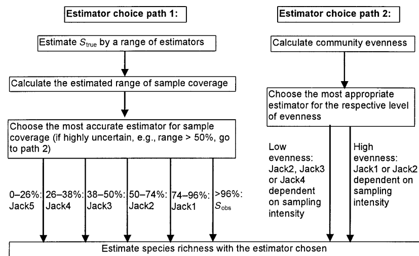
FIGURE 3.1 – Arbre de décision du meilleur estimateur du nombre d'espèces, in Brose et al. a
