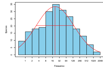
FIGURE 3.3 – Ajustement du modèle de Preston aux données de BCI.
