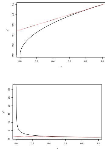
FIGURE 9.2 – Approximation de (\mathbf{Zp})_s^{q-1} par son développement limité au premier ordre pour q = 1.5 en haut ( r = q - 1 ) et q = 0.5 en bas.
