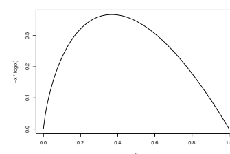
FIGURE 3.7 – courbe de -x \ln x entre 0 et 1.).
