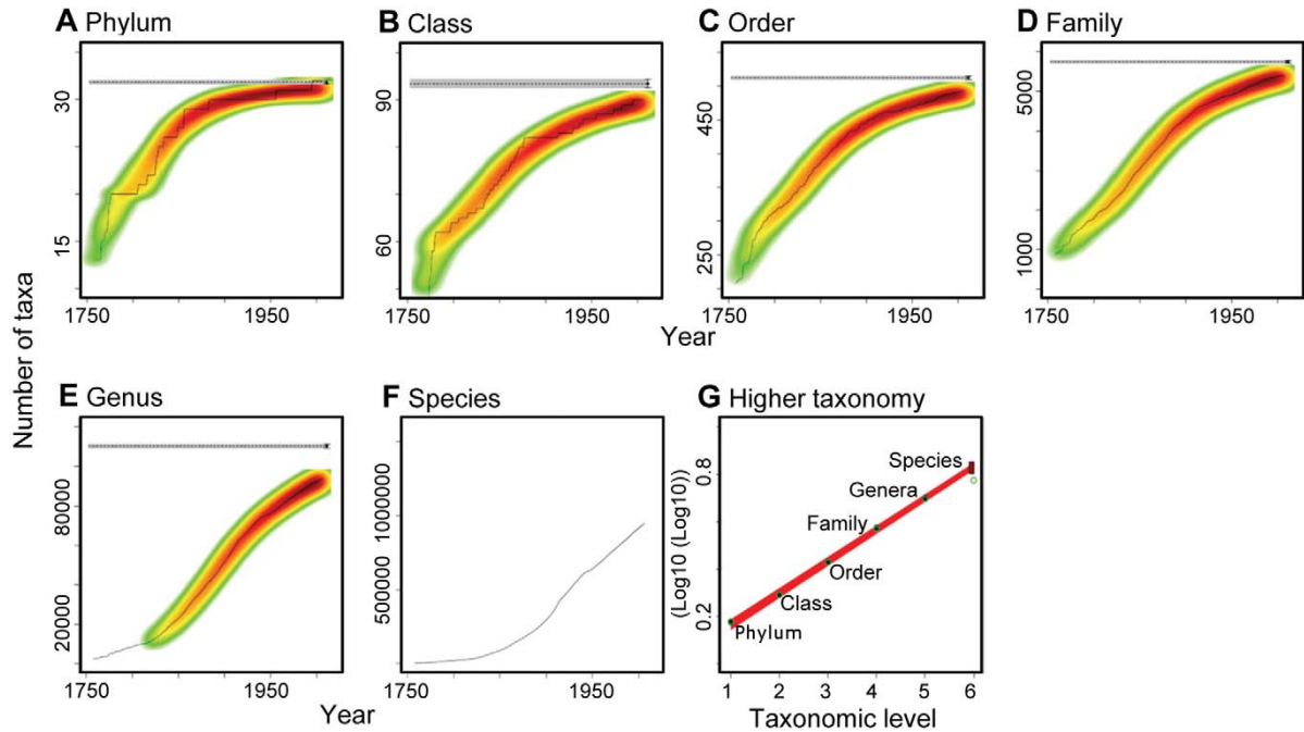
FIGURE 3.6 – Évolution du nombre de taxons connus en fonction du temps et valeur estimée du nombre total (ligne horizontale grise, A à E). Le nombre d'espèces connues est trop faible pour utiliser cette méthode (F). Il est obtenu par extrapolation de la relation du nombre de taxons d'un niveau à celui du niveau supérieur (G). In C. Mora et al. (2011). « How Many Species Are There on Earth and in the Ocean ? » In : PLoS Biol 9.8, e1001127, fig. 1, Animalia seulement.
