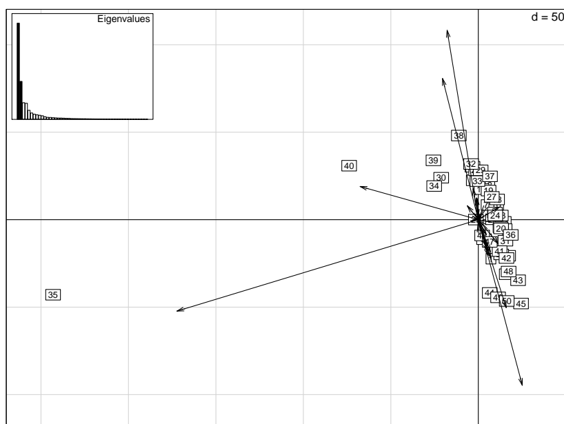
FIGURE 11.5 – ACP centrée des 50 carrés de BCI pour visualiser la diversité \beta .
