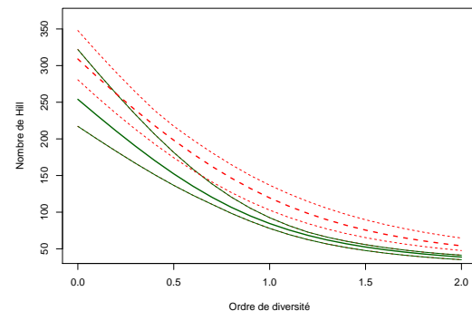
(b) Diversité HCDT. Les profils se chevauchent jusqu'à q \approx 0,7 .
