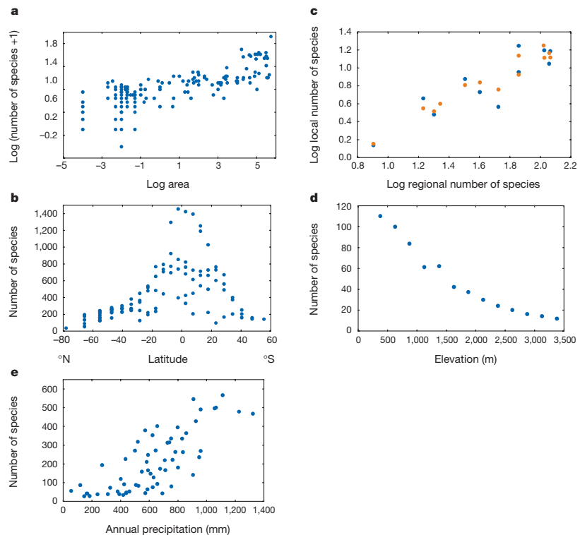
FIGURE 1.2 – Patrons de biodiversité. a (a) Le nombre d'espèces de vers de terre augmente en fonction de la surface échantillonnée, de 100 m 2 à plus de 500 000 km 2 selon la relation d'Arrhenius (voir page 210). (b) Nombre d'espèces d'oiseaux en fonction de la latitude. (c) Relation entre la richesse régionale et la richesse locale. (d) Nombre d'espèces de chauve-souris en fonction de l'altitude dans une réserve au Pérou. (e) Nombre d'espèces de végétaux ligneux en fonction des précipitations en Afrique du Sud
