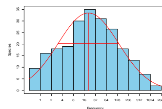
FIGURE 3.3 – Ajustement du modèle de Preston aux données de BCI.
