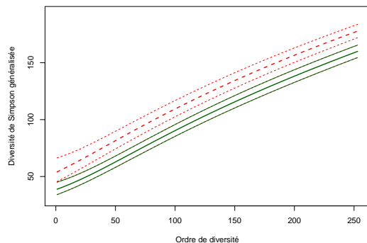
(a) Diversité généralisée de Simpson (nombres effectif d'espèces). Les profils sont distincts, ce qui permet de conclure que la parcelle 6 est plus diverse que la parcelle 18.
